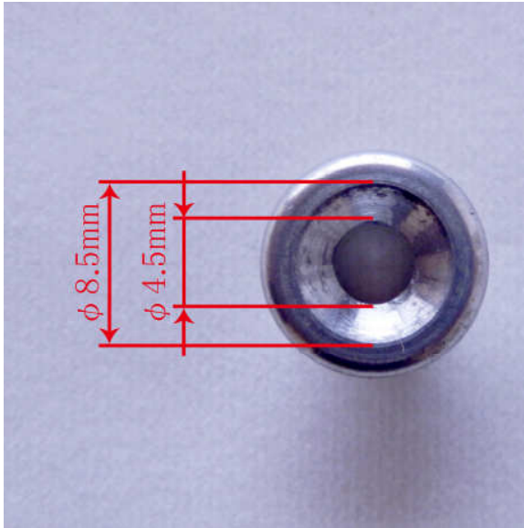
図 1 上面図
