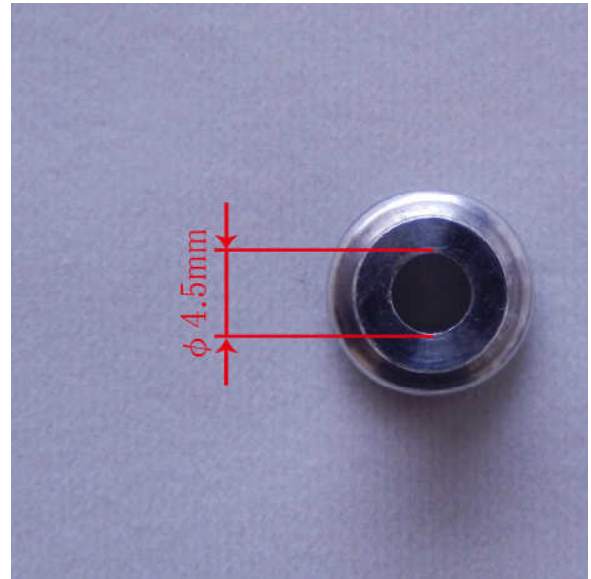
図 2 下面図
